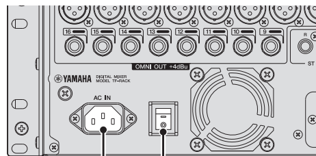
电源开关 交流电源输入
