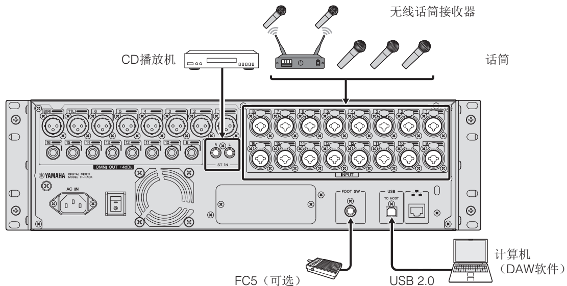
各通道的默认信号路径
